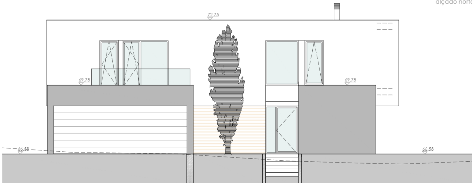
alçado poente
